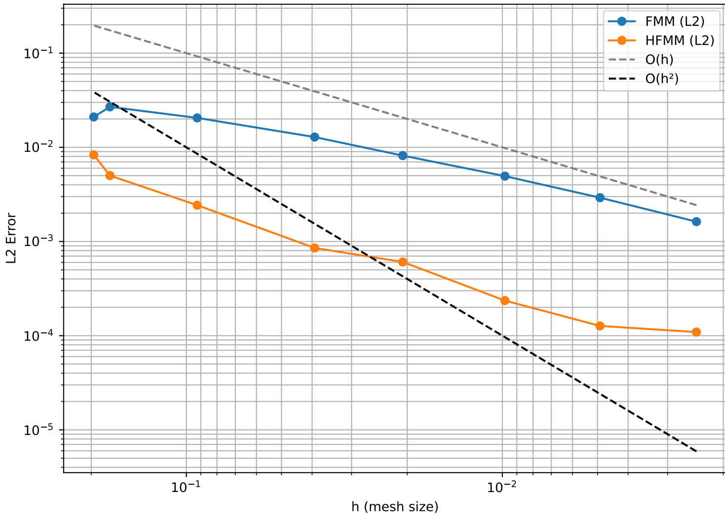
FMM Convergence - L-Cylinder
